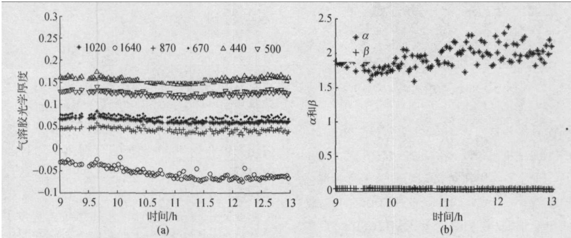
图 4 2007-10-12 大气气溶胶光学特征 (a) 各通道气溶胶光学厚度随时间变化; (b) 波长指数( \alpha )和浑浊系数( \beta )
